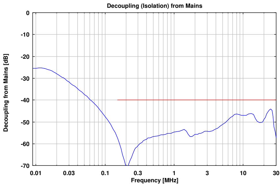
Abb. 8 Entkopplung vom Speisnetz Fig. 8 Decoupling from mains
